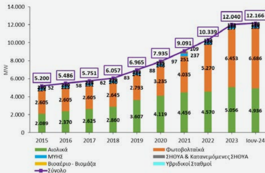
Διάγραμμα 114: Εξέλιξη εγκατεστημένης ισχύος στο σύνολο της Επικράτειας ανά τεχνολογία ΑΠΕ (MW), 2015 – Ιούνιος 2024
