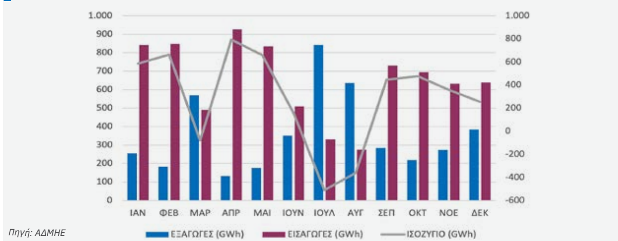
Διάγραμμα 82: Εξέλιξη φυσικών ροών ενέργειας 2022
