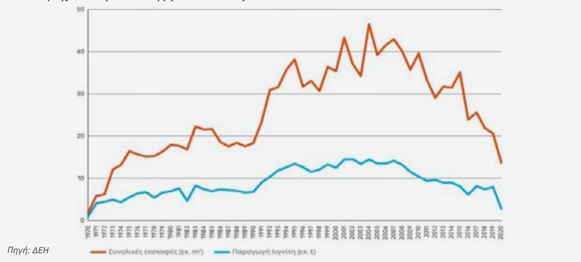
Διάγραμμα 107: Διαχρονική εξέλιξη παραγωγής λιγνίτη και συνολικών εκσκαφών στα ορυχεία Μεγαλόπολης (1970 – 2020)
