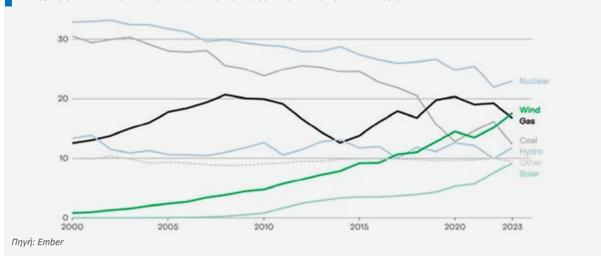
Διάγραμμα 15: Μεριδίο ηλεκτροπαραγωγής στην ΕΕ (%), ανά πηγή
