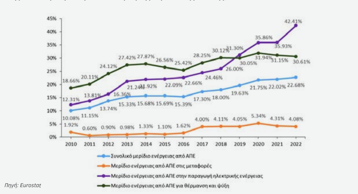
Διάγραμμα 108: Συνολικά και Ειδικά Μερίδια Συμμετοχής των ΑΠΕ Στο Ενεργειακό Σύστημα της Ελλάδας στη Βάση Μεθοδολογίας της Ευρωπαϊκής Ένωσης, 2010-2022
