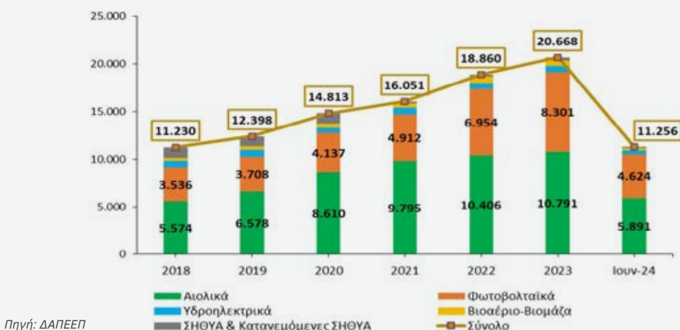
Διάγραμμα 110: Εξέλιξη παραγωγής ενέργειας από ΑΠΕ ανά τεχνολογία στο Διασυνδεδεμένο Σύστημα (GWh), 2018 – Ιούνιος 2024
