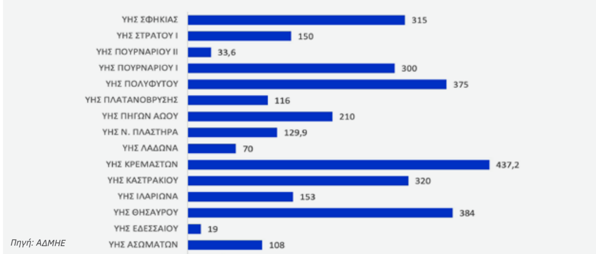
Διάγραμμα 130: Καθαρή ισχύς Υδροηλεκτρικών Σταθμών στην Ελλάδα (MW), Δεκέμβριος 2023
