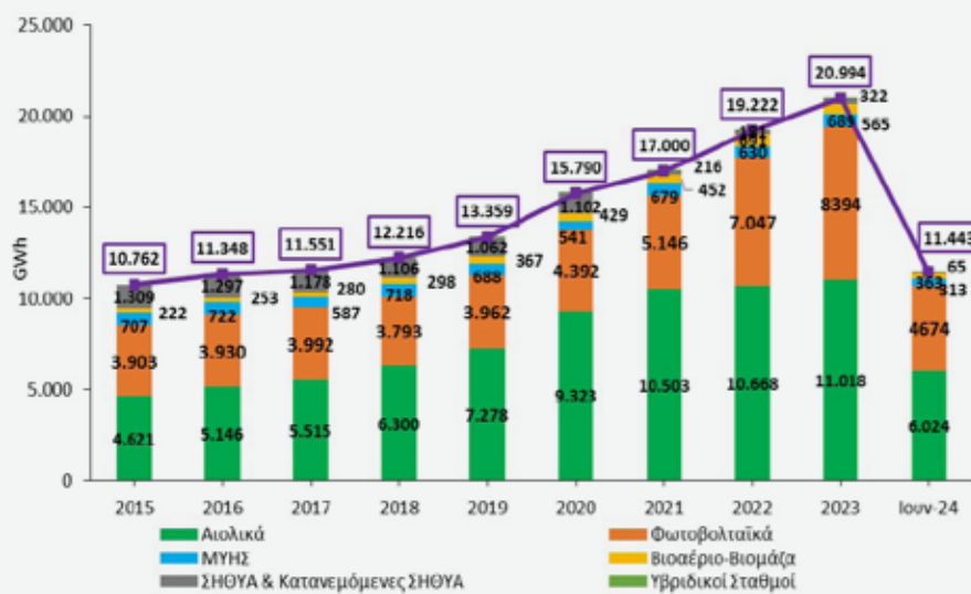
Διάγραμμα 111: Εξέλιξη παραγωγής ενέργειας ανά τεχνολογία ΑΠΕ (GWh) στο σύνολο της Επικράτειας, 2015- Ιούνιος 2024
