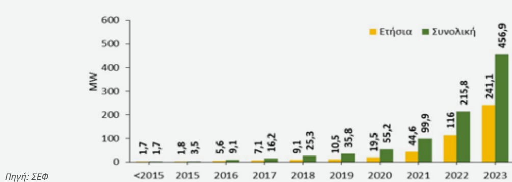
Διάγραμμα 123: Ετήσια και συνολική εγκατεστημένη ισχύς φωτοβολταϊκών συστημάτων αυτοκατανάλωσης, 2015-2023
