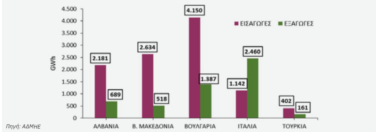
Διάγραμμα 83: Εμπορικά προγράμματα εισαγωγών-εξαγωγών ηλεκτρικής ενέργειας ανά διασύνδεση της Ελλάδας το 2023 (GWh)
