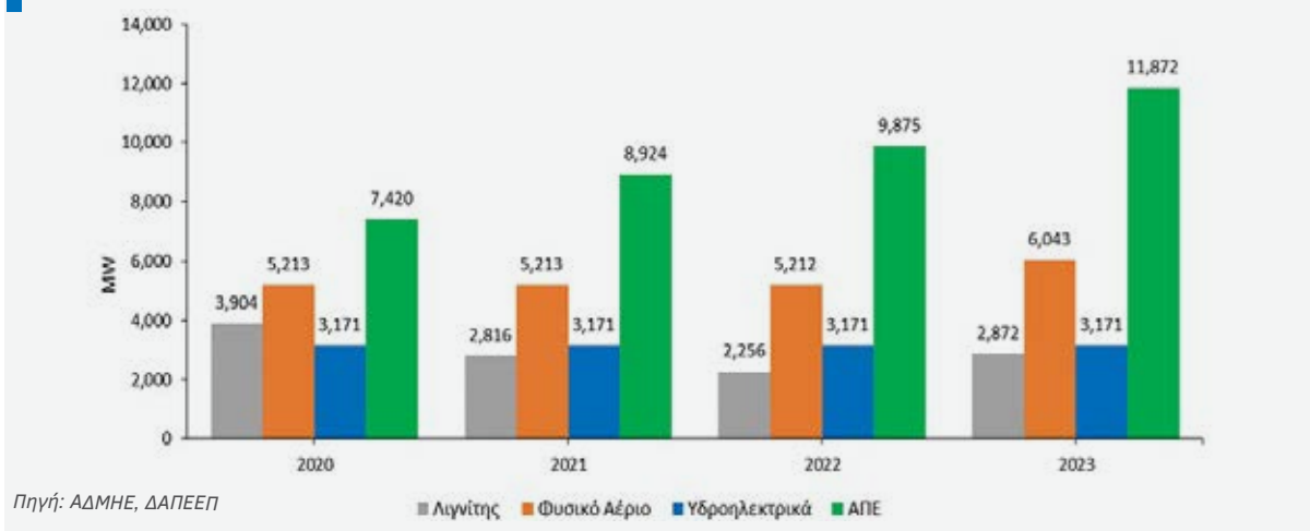
Διάγραμμα 80: Συνολική Εγκατεστημένη Ισχύς Μονάδων ανά Καύσιμο 2020-2023
