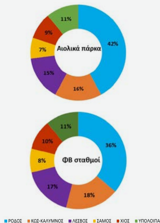
Διάγραμμα 134: Γεωγραφική κατανομή εγκατεστημένης ισχύος ΑΠΕ στα Μη Διασυνδεδεμένα Νησιά, Απρίλιος 2024
