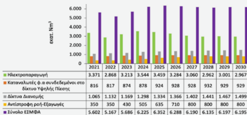
Διάγραμμα 60: Εκτίμηση Ζήτησης Φυσικού Αερίου στην Ελλάδα βασικού σεναρίου – ΕΣΕΚ adjusted, 2021-2030
