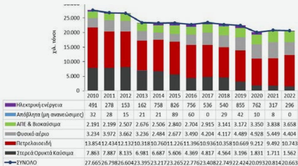
Διάγραμμα 28: Εξέλιξη Συνολικής Προσφοράς Ενέργειας στην Ελλάδα ανά πηγή (ktoe), 2010-2022
