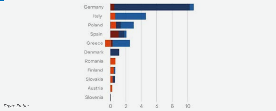
Διάγραμμα 14: Κλείσιμο ανθρακικών μονάδων για ηλεκτροπαραγωγή στην ΕΕ (σε GW)
