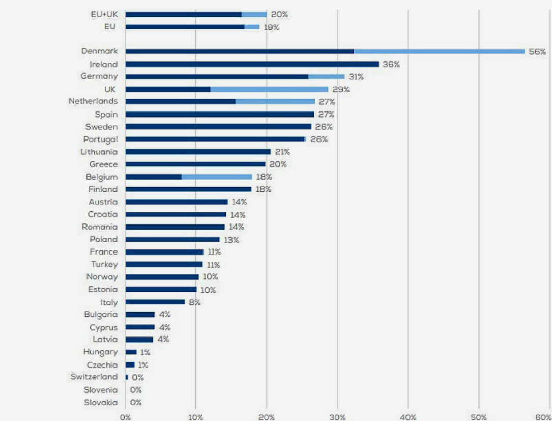
Διάγραμμα 120: Ποσοστό ηλεκτρικής ζήτησης που καλύπτεται από αιολική ενέργεια το 2023 σε διάφορες χώρες της Ευρωπαϊκής Ένωσης
