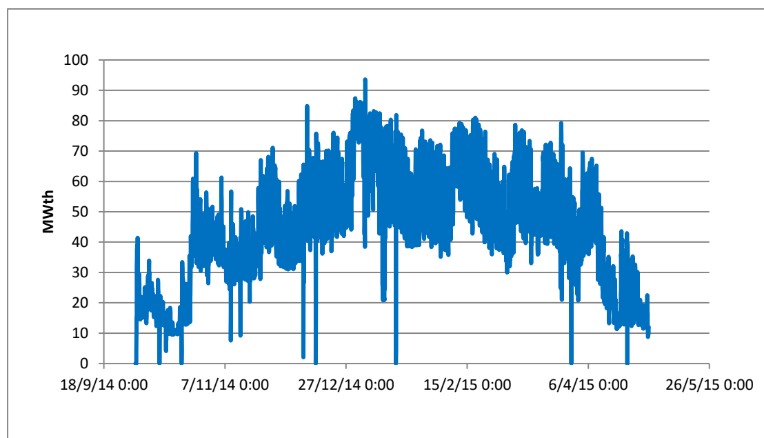
Διάγραμμα 13 - Κατανομή Συνολικής Ωριαίας Ζήτησης της Θερμικής Ενέργειας στην T/Θ Πτολεμαΐδας, 2014-2015
