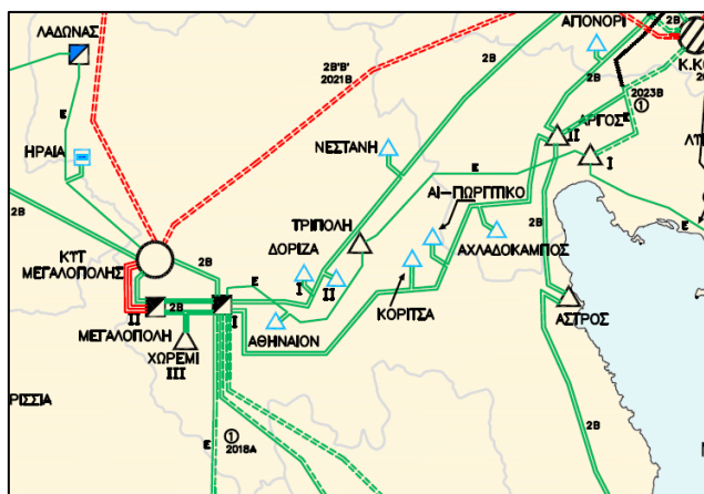
Χάρτης 9 – Υποδομές Συστήματος Μεταφοράς Ηλεκτρικής Ενέργειας στην Λιγνιτική Περιοχή Μεγαλόπολης Αρκαδίας
