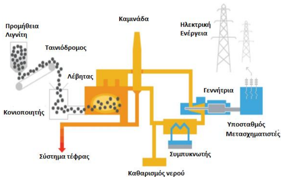
Διάγραμμα 10 – Σχηματική Απεικόνιση Λειτουργίας Λιγνιτικού ΑΗΣ Παραγωγής Ηλεκτρικής Ενέργειας
