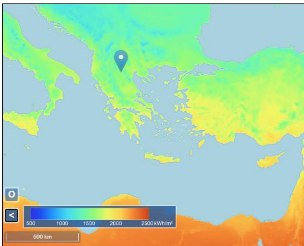
Χάρτης 11 - Ηλιακό Δυναμικό Ελλάδας – Μέση Ετήσια Προσπίπτουσα Ηλιακή Ακτινοβολία στο Οριζόντιο Επίπεδο
